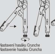
Nastavení hasáku Crunch Nastavenie hasáku Cruncha
